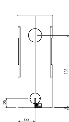
背面図
