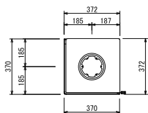
平面図
