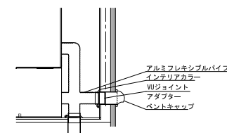
外気導入取付図
