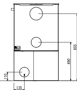
背面図
