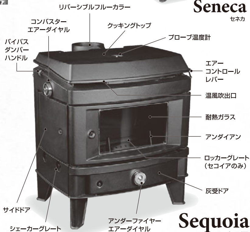
ダンパー閉じる
