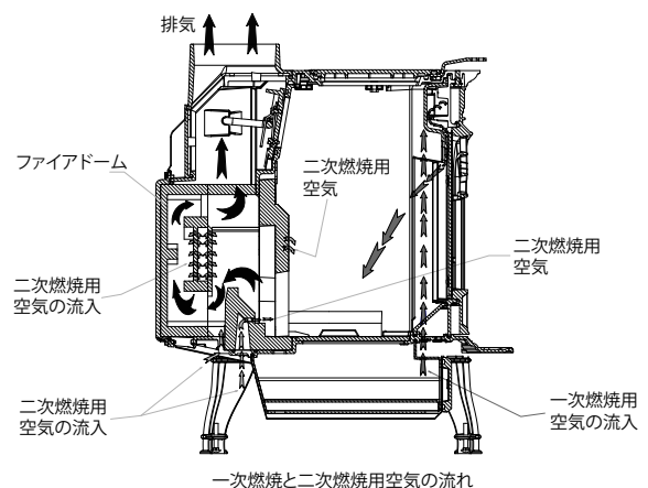
一次燃焼と二次燃焼用空気の流れ
