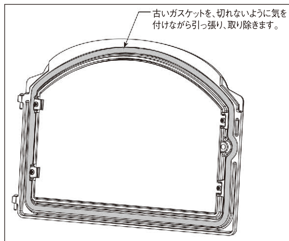
図14 ドアガasket
